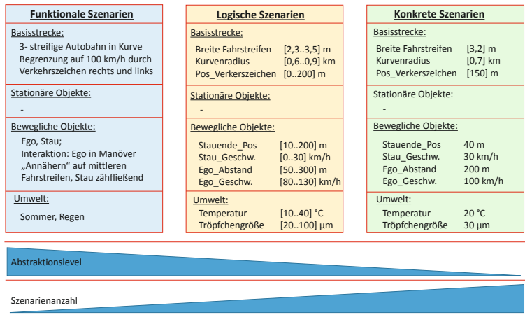
Abbildung 2: Abstraktionsebenen von Szenarien anhand eines Beispielszenarios im Entwicklungsprozess nach Norm ISO 26262
